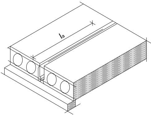
Figur 7.3.1/2 Armeringsføring ved længdefuge/randfuge
